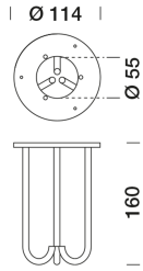
8950030 Tie-rod Ø 114 mm x D. 160 mm
