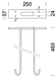
8950070 Tie-rod L. 250 x D. 57 x H. 460 mm
