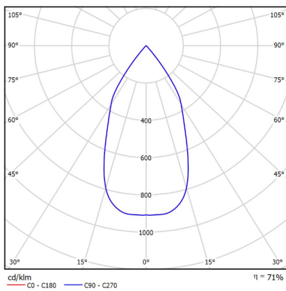
31W Óptica 54° / 54° Optics
